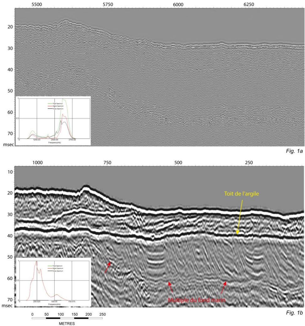
Figure 1 : Comparaison d'un profil acquis au SBP (Pinger 3.0 khz) et en sismique 2D multi-traces (airgun,5 ci)
