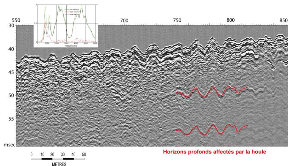
Figure 3 : Exemple d'acquisition sparker monotrace (sparker 150 J, 8 canaux espacés de 1 et directement sommés en 1). En profondeur on voit que tous les marqueurs sont affectés par des ondulations en phase, qui sont liées à la houle ou aux vagues.
