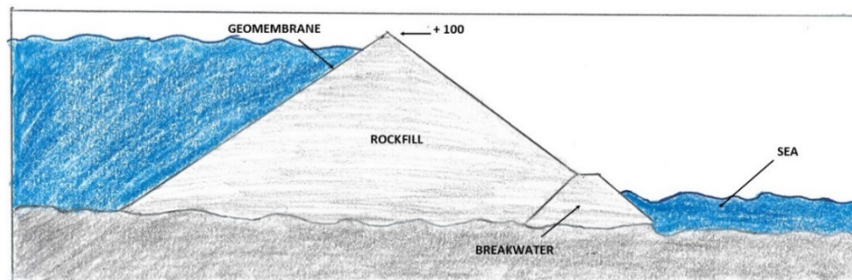
Fig. 2. Rockfill.
